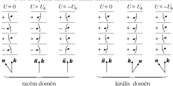
6. ábra. B_2 -fázis racém és királis tartományainak szerkezete
