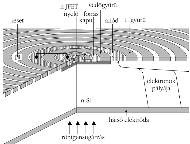
1. ábra. A szilícium drift dióda vázlat
