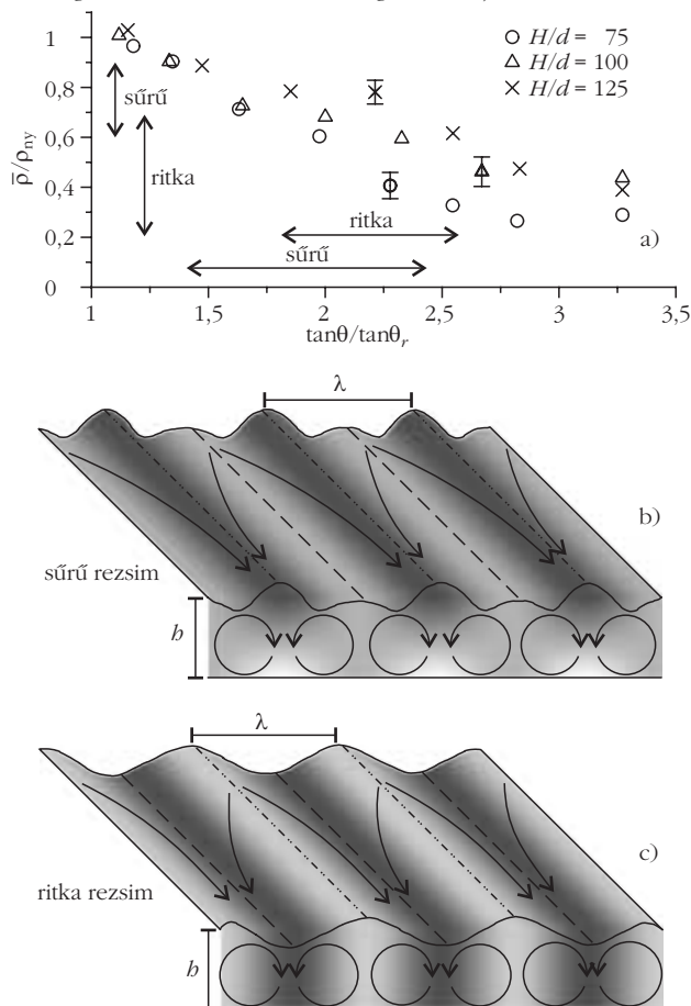
5. ábra. (a) A nyugalmi sűrűséggel ( \rho_{ny} ) normált átlagos anyagűrűség a meredekség függvényében három különböző H/d értékre. Az áramlási tér sematikus ábrája a sűrű (b) és ritka (c) rezsimekben. A sűrűség térbeli változását a szürkesség mértéke jelöli.
