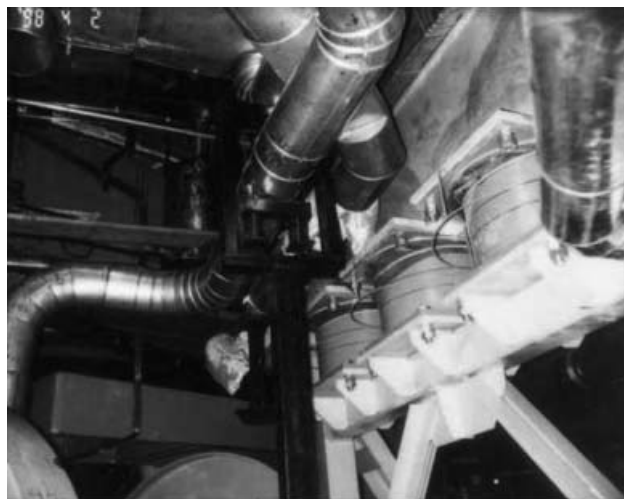
1. ábra. Viszkózus lengéscsillapítók a gőzfejlesztők alatt.
