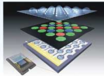
6. ábra. Színszűrők és mikrolencsék a színes képhez és a fényérzékenység növeléséhez
