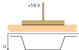
3. ábra. Feszültségeloszlás a pixel belsejében
