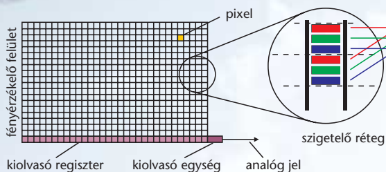
4. ábra. Négyzetrácsos elrendezés a tartalom kiolvasásához
