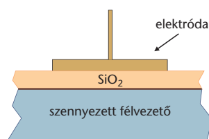
1. ábra. Egy pixel szerkezete
