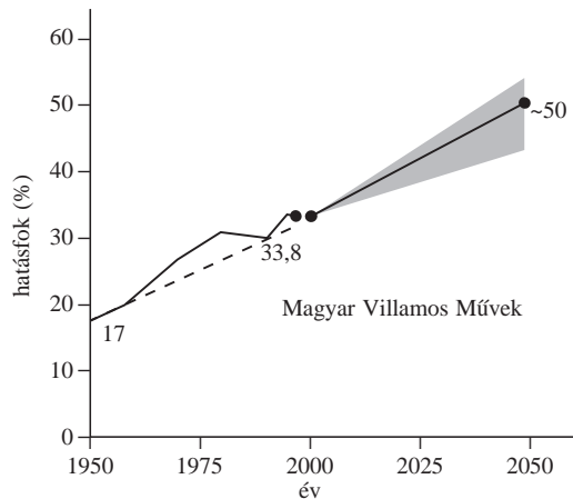
9. ábra. A villamosenergia-termelés hatásfoka Magyarországon 1950 és 2050 között [8]
