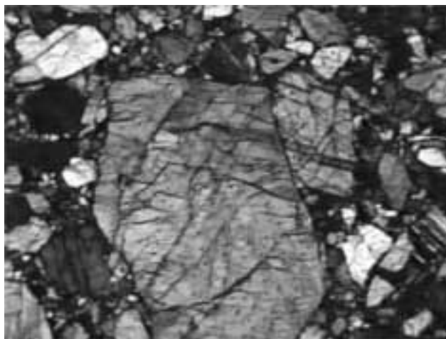
3. ábra. Anortozitminták a NASA-készletből: a 60025 számú kőzetminta részlete.
