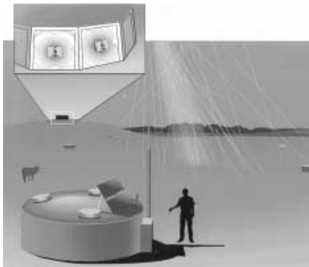
3. ábra. Plakátszerű ábrázolás az argentinai Pierre Auger Kozmikus Sugárzási Observatórium bemutatására. A Cserenkov-tartály mellett egy magaslat tetején kinagyítva ábrázolja az atmoszférára irányított fotodetektorokat, amelyek észlelik a záporbeli ütközésekkel gerjesztett légköri atomok, molekulák lumineszcens fénykibocsátását. A két észlelés megnövelt biztonsággal rekonstruálja a zápor kifejlődésének téridő-szerkezetét.
