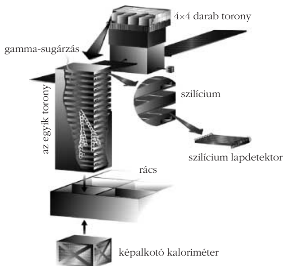
4. ábra. A LAT-detektor felépítése és működési elve
