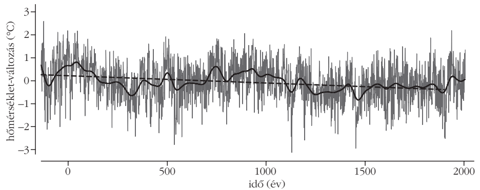
2. ábra. A németországi nyári hőmérséklet bő 2000 éves változása a fák évgyűrűiből [2].
