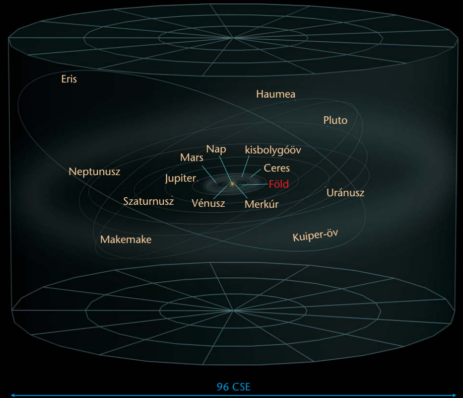
Naprendszer
