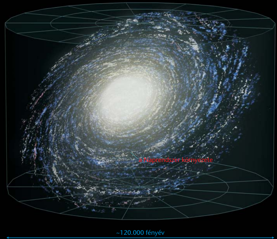
A Tejútrendszer
