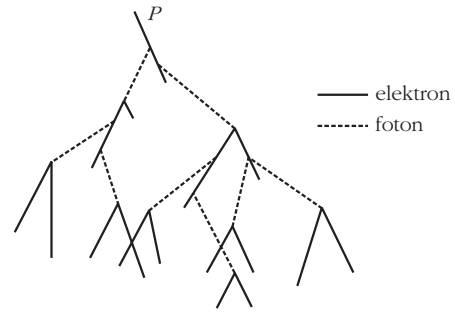
3. ábra. Az elektron-foton kaszkádzápor kifejlődésének vázlatos képe [2]. A kihúzott vonalak az elektronok, a szaggatott vonalak a fotonok nyomait jelzik. A rajzon a P primer elektron útközben fotonokat vált ki, a fotonok viszont egy-egy elektron-positron párt keltenek, és így tovább. A Wilson-féle ködkamrában csak az ionizáló elektronok és pozitronok nyomai láthatók, a fotonoké nem.
