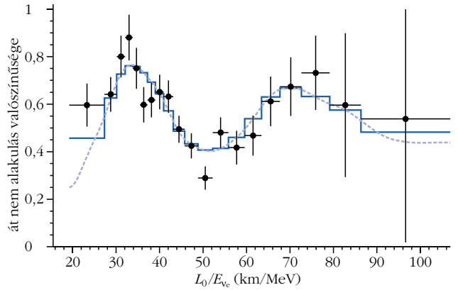
13. ábra. Az át nem alakulás valószínűsége az ízrezgés elmélete szerint (folytonos vonal), összevetve a Daya-Bay kísérletben mért adatokkal (pontok a bizonytalanságot jellemző vonalakkal).
