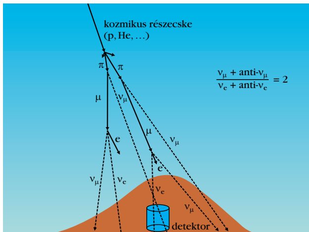
7. ábra. Koszmikus részecske által a légkör felső rétegében keltett részecskeszópor vázlatos rajza.
