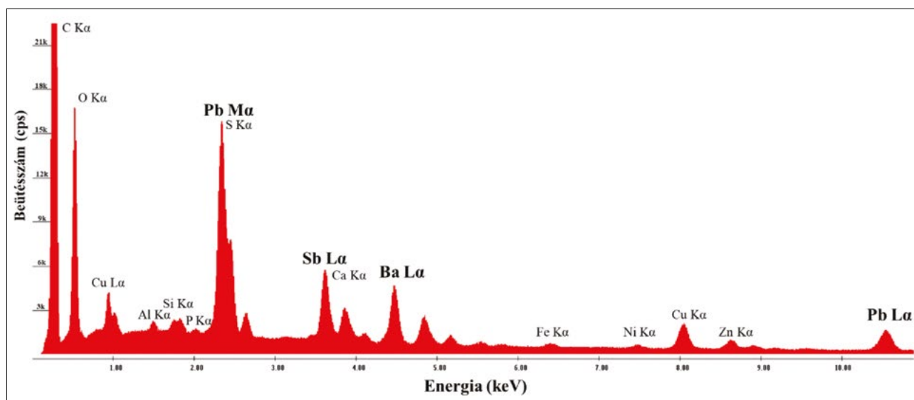
4. ábra. Egy karakterisztikus, ún. három komponensű lőmaradvány-szemcse tipikus röntgenspektruma, melyen jól láthatók az ólom, az antimon és a bárium, továbbá a másodlagos kémiai elemeknek megfelelő csúcsok. A görbe alatti terület – a módszer félkvantitatív jellegéből adódóan – az adott kémiai elem relatív koncentrációjáról ad információt
