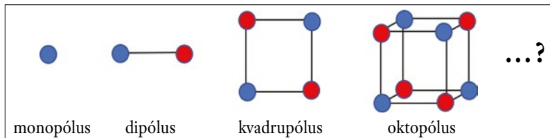
2. ábra. Az inhomogén töltéeloszlás lehetséges közelítései atommagokra. A piros és kék körök ellentétes töltések parciális szeparálódását jelképezik
