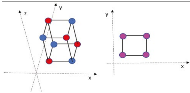
4. ábra. A háromdimenziós koordináta-rendszer célszerű elforgatása egy téglalap lehetséges legegyszerűbb leírása érdekében
