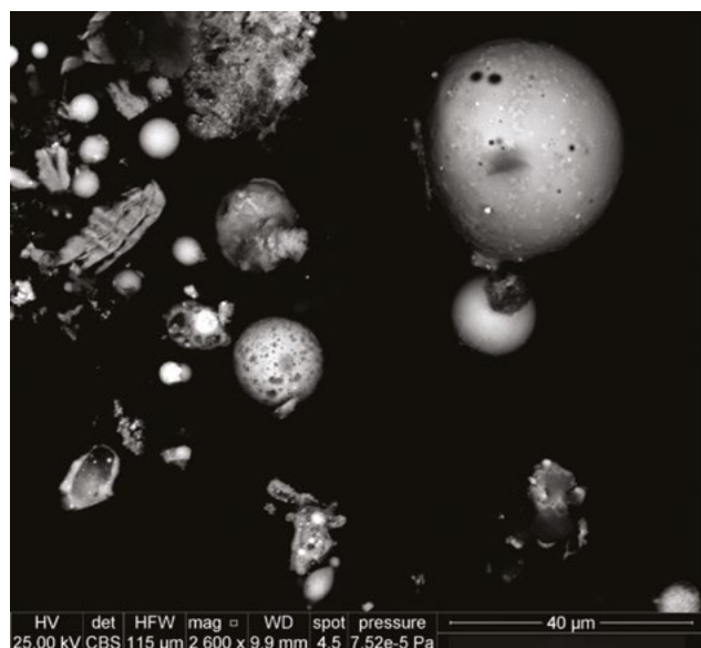
3. ábra. A visszaszórt elektronképen jellegzetes, gömb alakú lőmaradvány-szemcsék láthatók, melyek átmérője 1 és 30 \mu\text{m} közé esik
