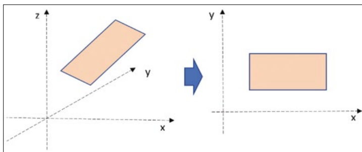
3. ábra. A háromdimenziós koordináta-rendszer célszerű elforgatása egy téglalap lehetséges legegyszerűbb leírása érdekében
