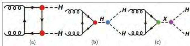
6. ábra. Higgs-bozonpár keletkezésének lehetséges módjai a gluon-gluon fúzióban (a gluon az ütköző proton alkotórésze). A harmadik lehetőség a standard modell valósskalár-kiterjesztésében lehetséges
