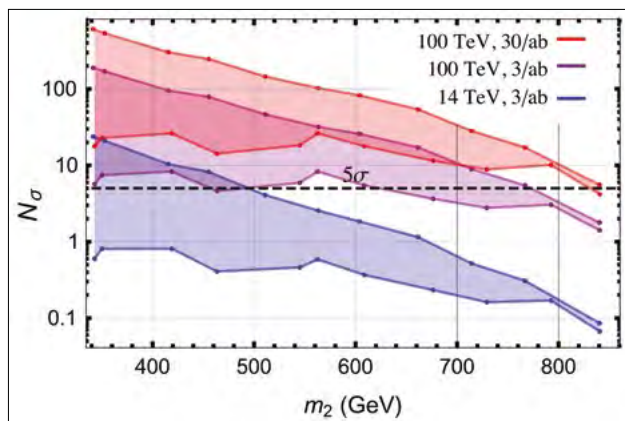
7. ábra. Egy új skalár részecskével (S) bővített standard modellben az S \rightarrow HH két Higgs-részecskét adó folyamat felfedezésének várható szignifikanciája az új részecske tömegének függvényében a HL-LHC-n és az FCC-hh gyorsítón különböző adatmennyiségek feldolgozása után. A színes területek jelölik a megengedett paramétertartományt
