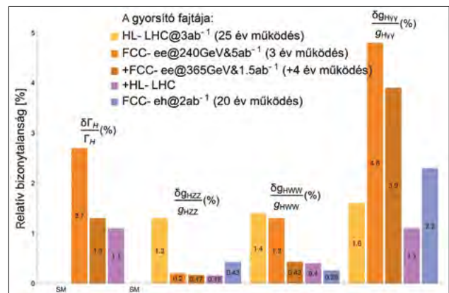
3. ábra. A Higgs-részecske teljes bomlási szélessége ( \Gamma_H ), valamint a Higgs-vektorbozon csatolások ( g_{HVV} , V = Z, W, \gamma ) mérésének várható relatív bizonytalansága a különböző jelenlegi és tervezett gyorsítók adatainak feldolgozásával. Ha a mérés nem kivitelezhető érdemlegesen az adott gyorsítón, akkor az „SM” jelzést alkalmaztuk, ami a standard modell elméleti becslésre utal, kísérleti bizonytalanság nélkül
