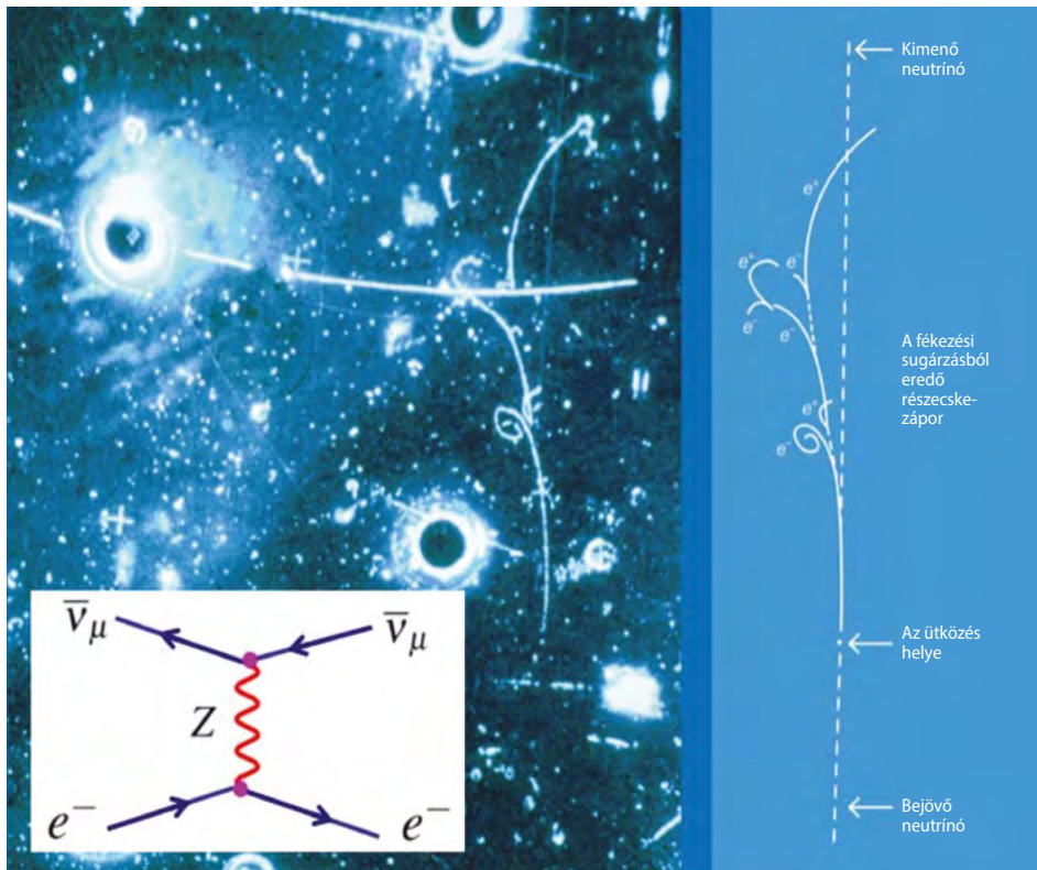
2. ábra. A beérkező anti-müon neutrínó kölcsönhatásba lép egy atomi elektronnal, és kilöki azt, egy elektro-mágneses záport elindítva így [11]
