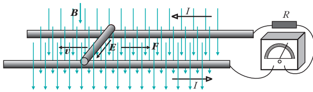
2. ábra. A Lenz-törvényre vezető gondolkísérlet [2].
