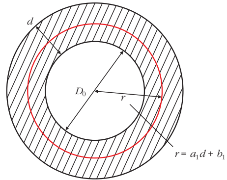
12. ábra. Állandó belső átmérőjű, változó falvastagságú rézcső keresztmetszetének vázlatos rajza.
