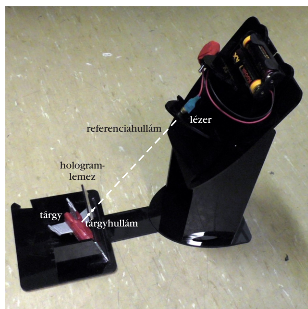
3. kép. A reflexiós hologram felvételi elrendezése.
