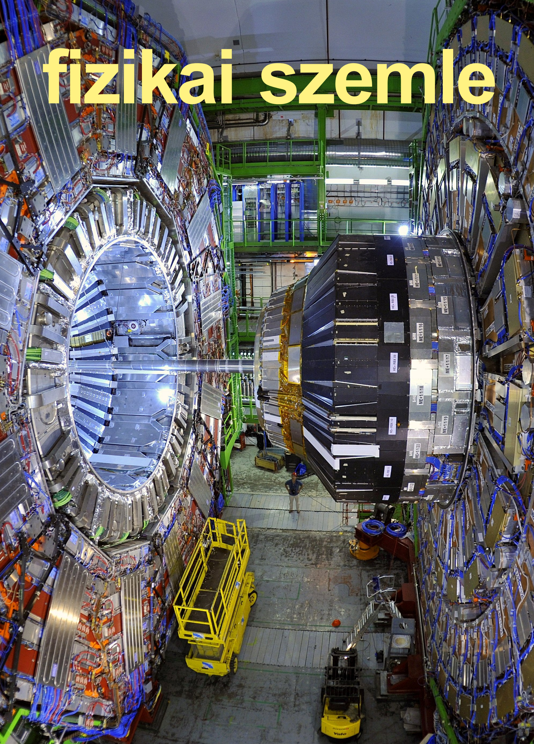
A CMS-detektor lezáró sapkája kihúzva. A dugórész elemei jelentős hazai részvétellel készültek. (2021. március)
