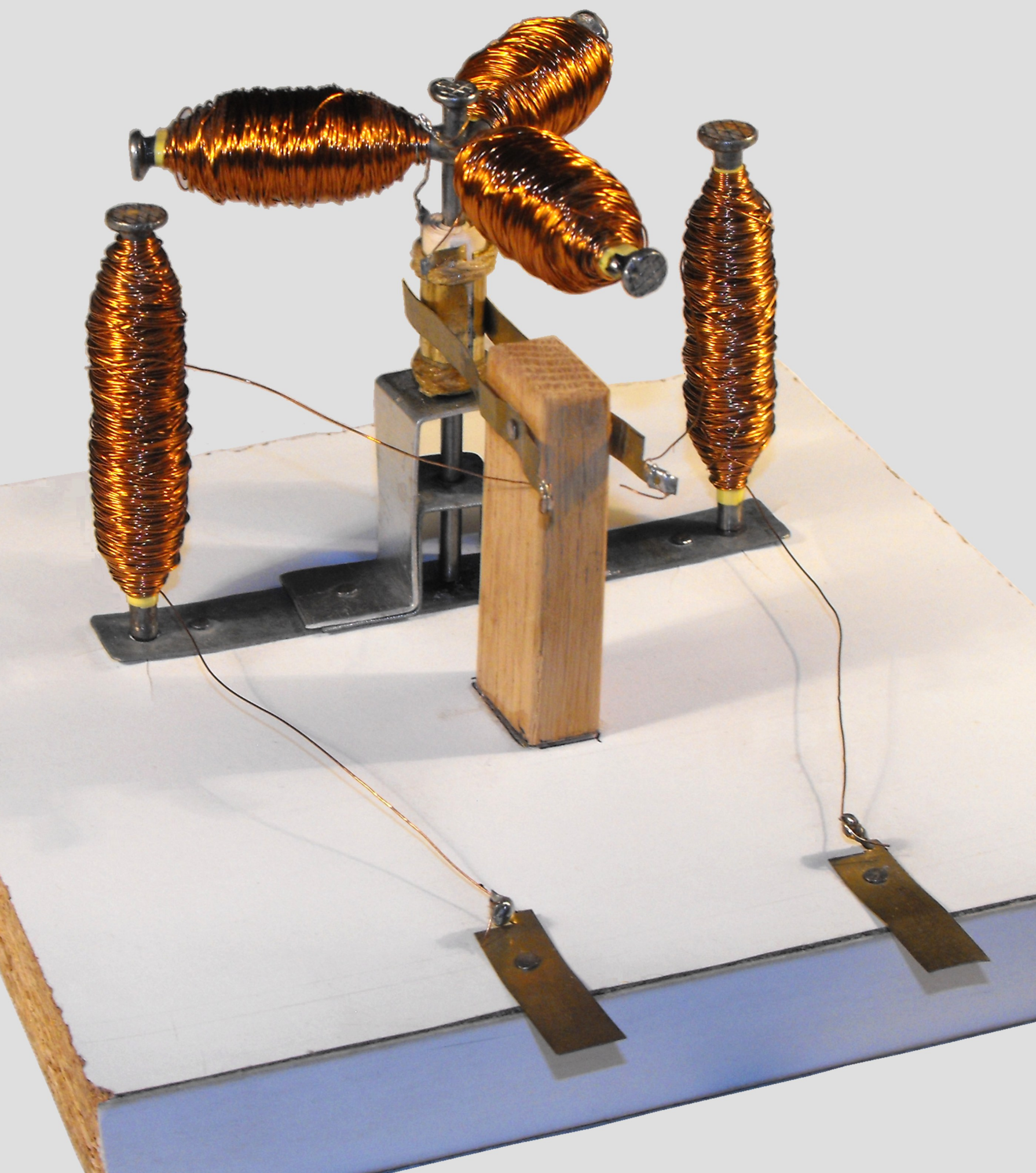
Egy jól sikerült, könnyen forgó szegmotor. (2021. január)
