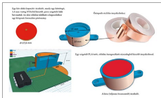
1. ábra. A 3D-nyomtatott detektor alkatrészei
