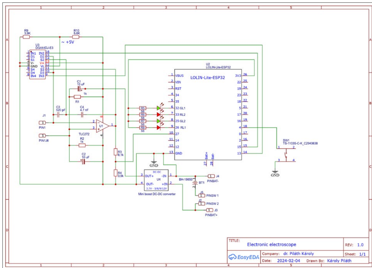
2. ábra. A töltésmérő részletes kapcsolási rajza
