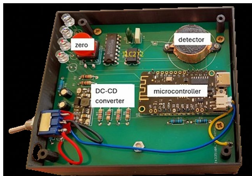
4. ábra. Az elkészült kísérleti példány fényképe
